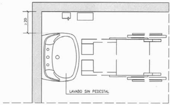
LAVABO ACCESIBLE
